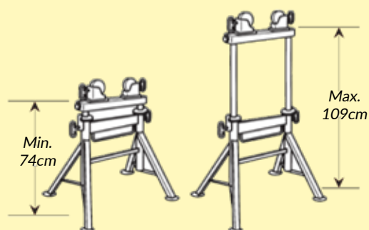
Pro Roll met stalen wielen
